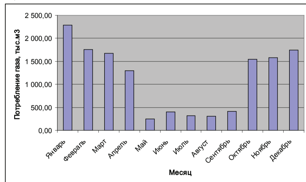
Рисунок 4 – потребление природного газа Первомайской ТЭЦ для выработки тепловой энергии для бойлерных в р.п. Первомайский за 2014 год
