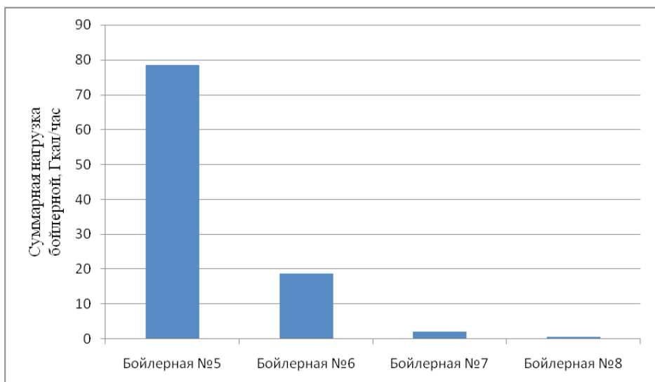
Гистограмма потребления тепловой энергии по бойлерным
