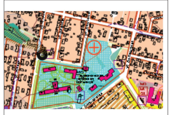
ПРЕДЛОЖЕНИЯ О ВНЕСЕНИИ ИЗМЕНЕНИЙ В ГЕНЕРАЛЬНЫЙ ПЛАН МО Р.П. ПЕРВОМАЙСКИЙ ЩЕКИНСКОГО РАЙОНА ТУЛЬСКОЙ ОБЛАСТИ СВОДНАЯ СХЕМА (ОСНОВНОЙ ЧЕРТЕЖ) ГЕНЕРАЛЬНОГО ПЛАНА ФРАГМЕНТ. М 1:5000
