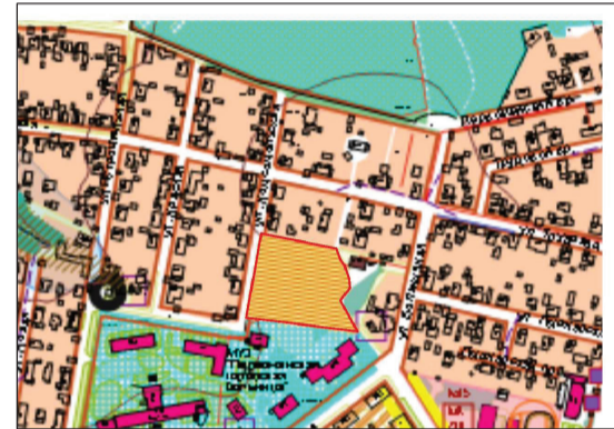
ПРЕДЛОЖЕНИЯ О ВНЕСЕНИИ ИЗМЕНЕНИЙ В ГЕНЕРАЛЬНЫЙ ПЛАН МО Р.П. ПЕРВОМАЙСКИЙ ЩЕКИНСКОГО РАЙОНА ТУЛЬСКОЙ ОБЛАСТИ СВОДНАЯ СХЕМА (ОСНОВНОЙ ЧЕРТЕЖ) ГЕНЕРАЛЬНОГО ПЛАНА ФРАГМЕНТ. М 1:5000
