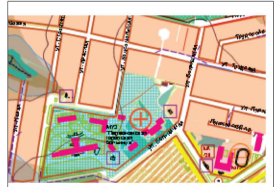
ПРЕДЛОЖЕНИЯ О ВНЕСЕНИИ ИЗМЕНЕНИЙ В ГЕНЕРАЛЬНЫЙ ПЛАН МО Р.П. ПЕРВОМАЙСКИЙ ЩЕКИНСКОГО РАЙОНА ТУЛЬСКОЙ ОБЛАСТИ СХЕМА ГРАНИЦ, ТЕРРИТОРИЙ, ЗЕМЕЛЬ И ОГРАНИЧЕНИЙ ГЕНЕРАЛЬНОГО ПЛАНА ФРАГМЕНТ. М 1:5000
