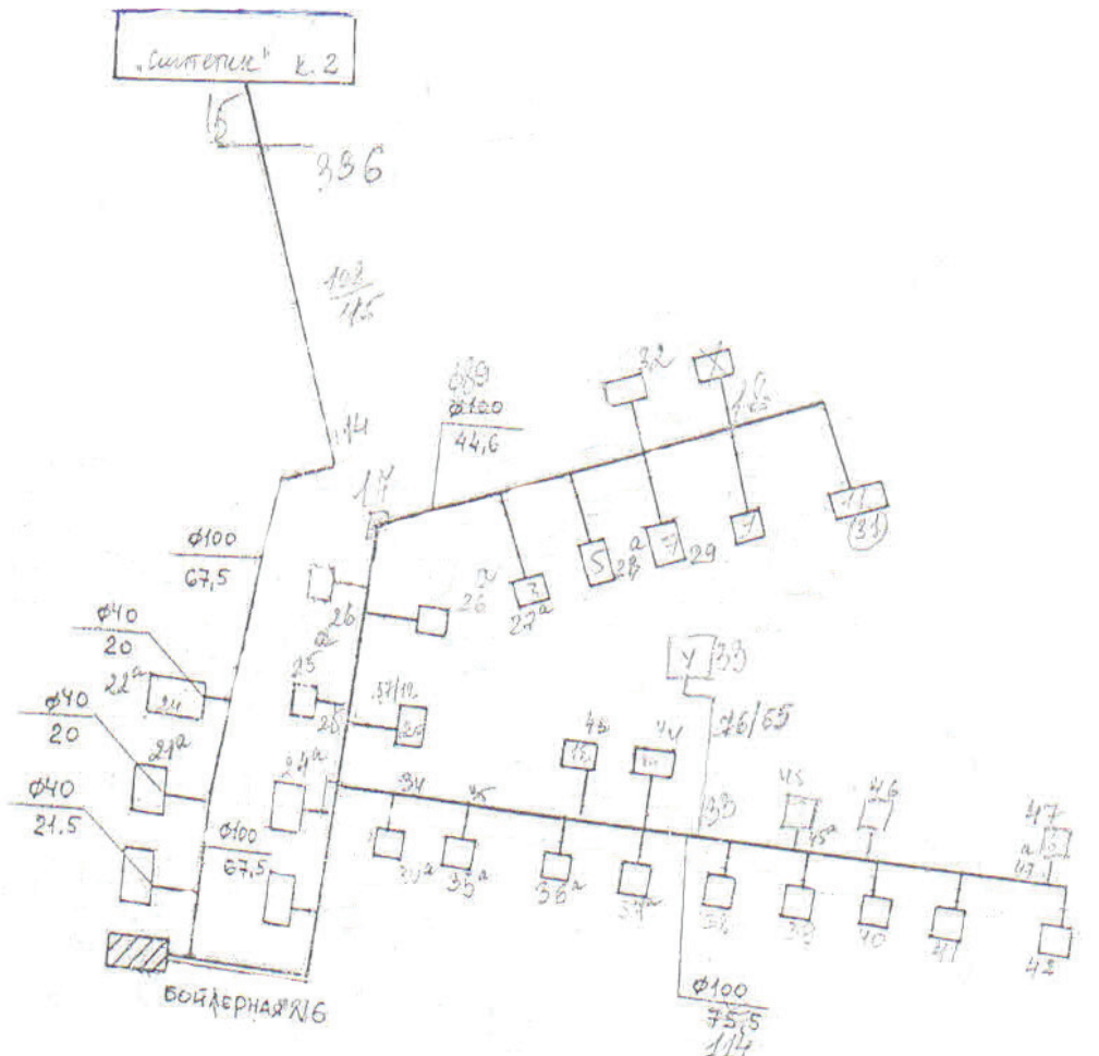
Рисунок 2 – Зона действия бойлерной №6
