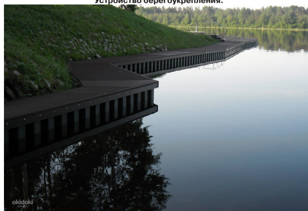
Устройство берегоукрепления.
